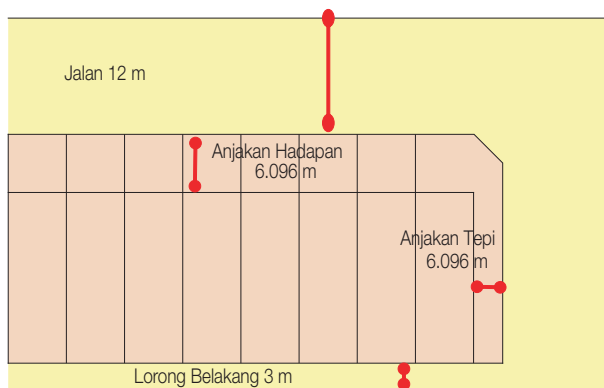
Anjakan bangunan bagi rumah teres
