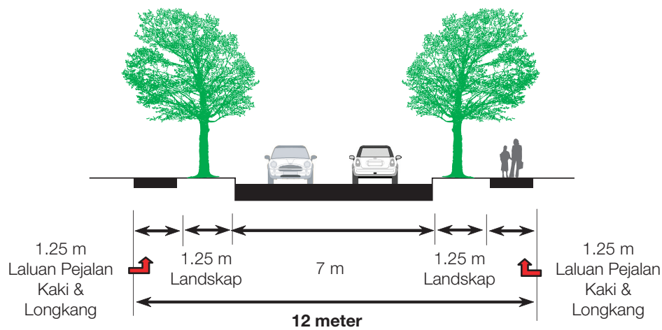
Keratan rentas jalan di dalam kawasan 'gated community'
